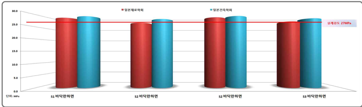
[그림 3.3.3] 반발경도법에 의한 비파괴강도 측정 결과-상부구조(바닥판하면)
