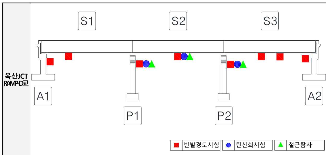
[그림 3.3.2] 비파괴시험 위치도
