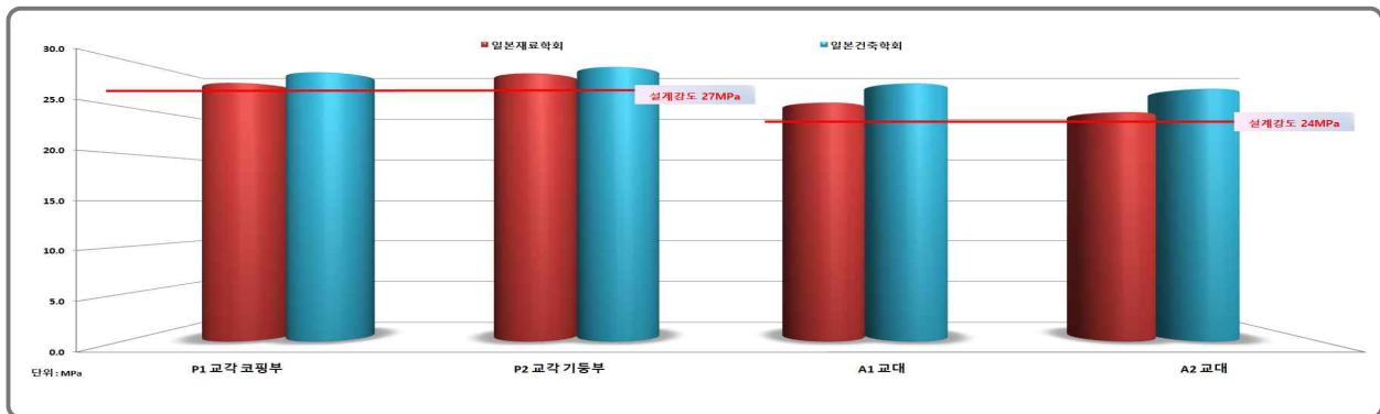
[그림 3.3.4] 반발경도법에 의한 비파괴강도 측정 결과-하부구조
